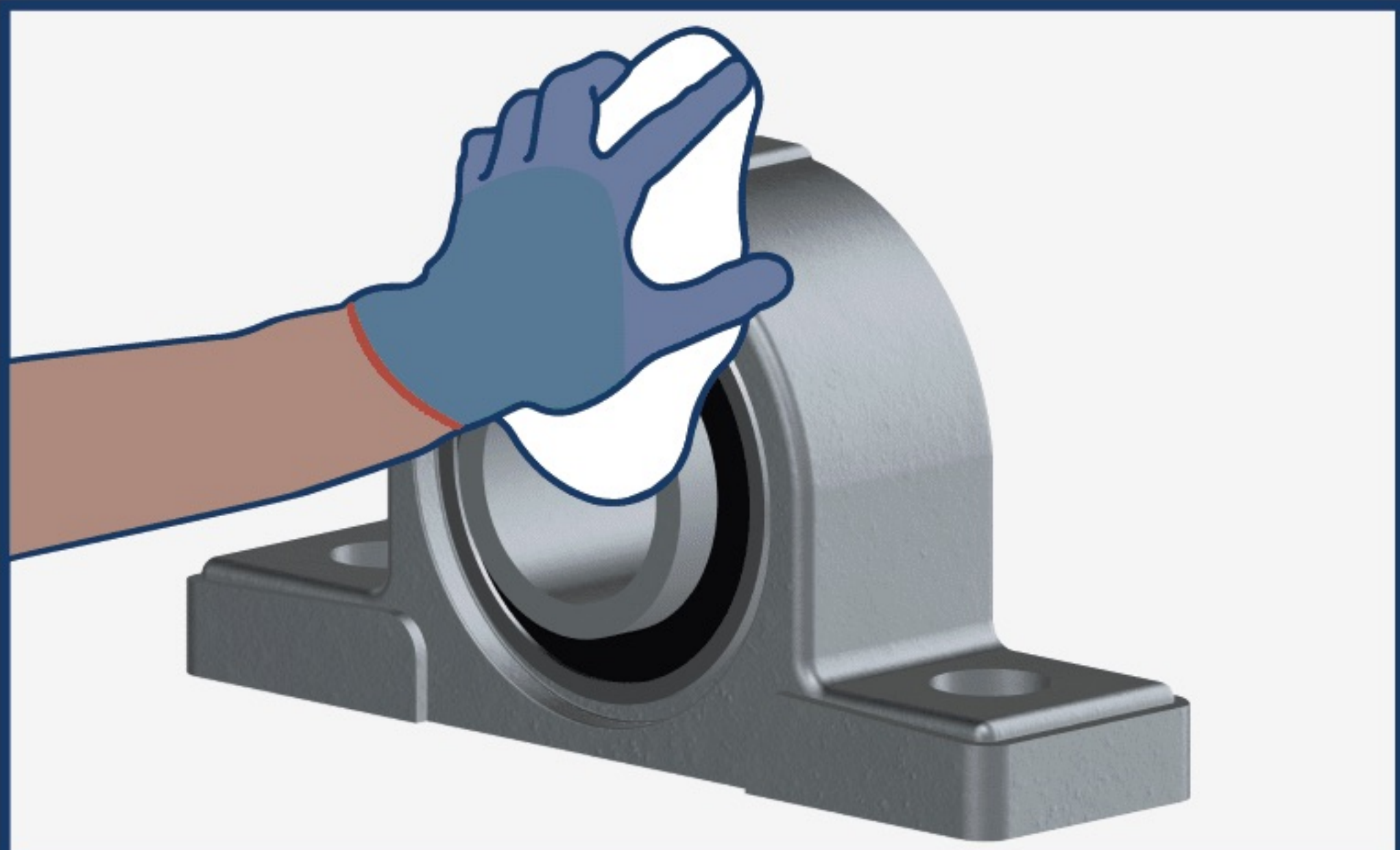
Reinigung der Schmierstelle
