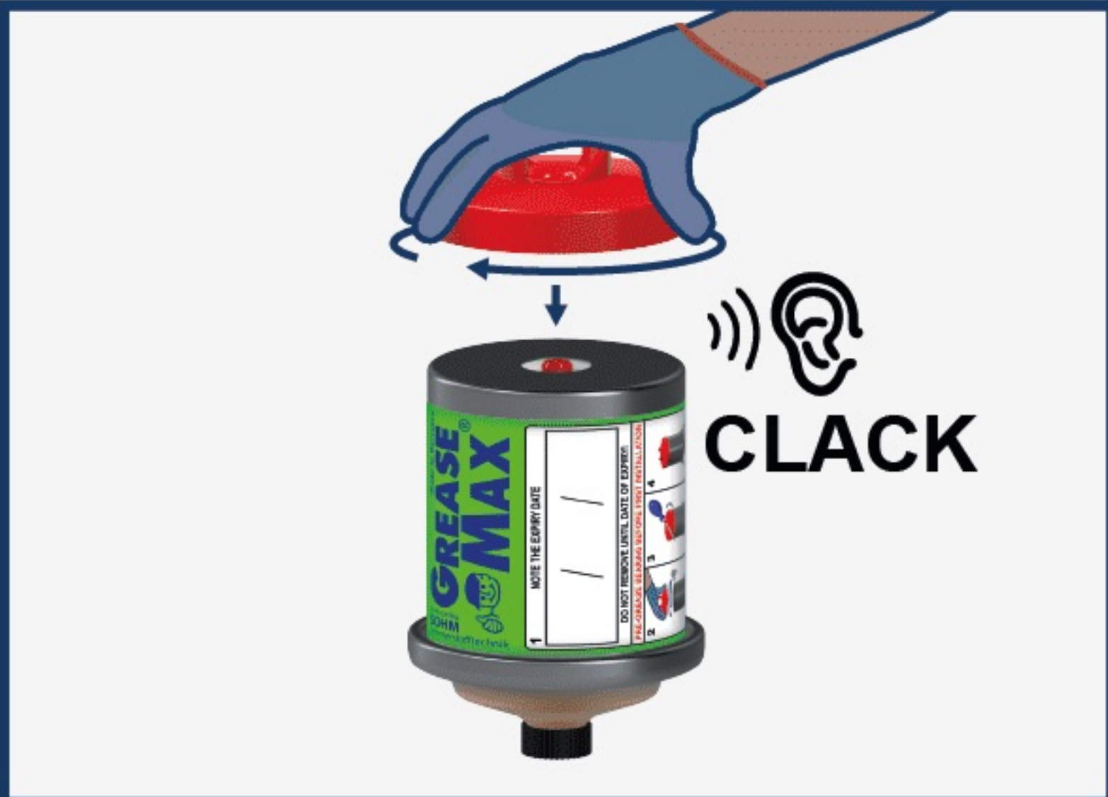
Startdeckel eindrehen, die Auslöseschraube dringt hörbar ein und weiterdrehen
